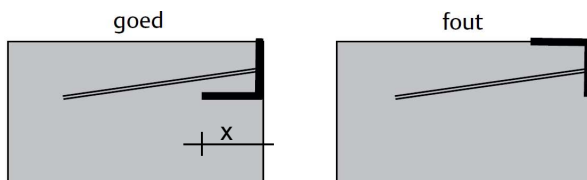
Figuur 2. Principe van een randbescherming.
